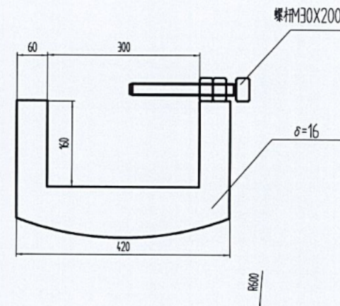
分流器夹具 材质：304不锈钢
